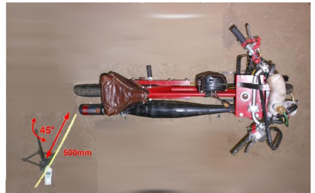
Illustration No2: Cas d'une machine avec l'échappement sur l'arrière :
